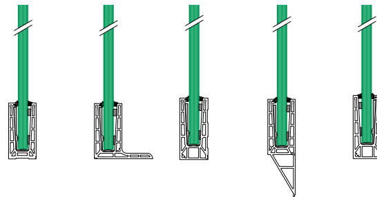
Easy Glass® Pro Topmontage / Ingieten Easy Glass® Pro F Topmontage Easy Glass® Pro Zijmontage Easy Glass® Pro Y Zijmontage Easy Glass® Pro Inverse Zijmontage
