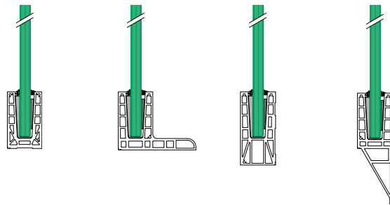
Easy Glass® Max Topmontage / Ingieten
