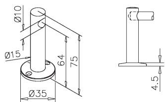
Eindsteun - 650 / 10
