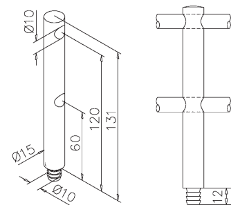
Dubbele middensteun - 666 / 10
