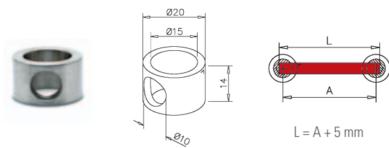
690 / 10 - voor eindsteun
