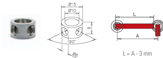
692 / 06 - voor hoeksteun 90°
