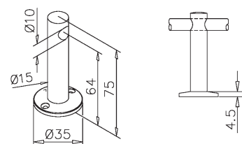
Middensteun - 651 / 10
