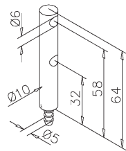
Dubbele eindsteun - 665 / 06
