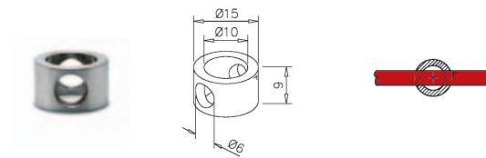
691 / 06 - voor middensteun
