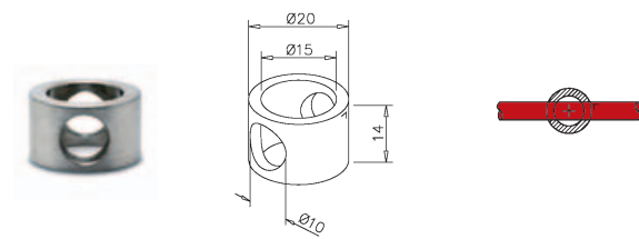
691 / 10 - voor middensteun
