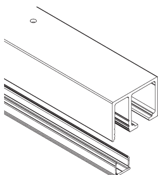
Railprofiel set met vast paneel, vorgeboord
