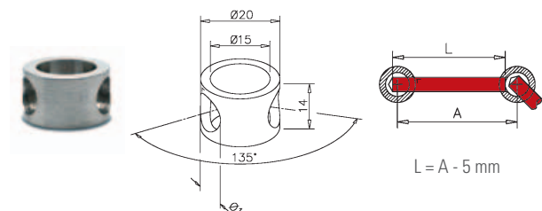
693 / 10 - voor hoeksteun 45°
