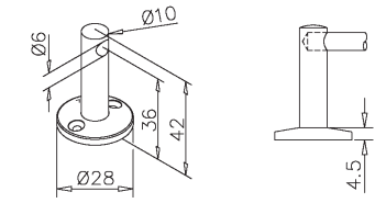
Eindsteun - 650 / 06
