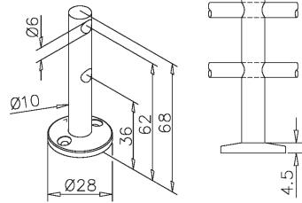
Dubbele middensteun - 656 / 06
