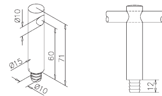
Middensteun - 661 / 10
