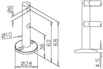
Dubbele eindsteun - 655 / 06
