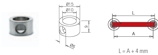
690 / 06 - voor eindsteun
