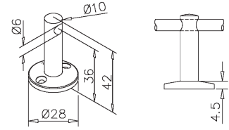
Middensteun - 651 / 06
