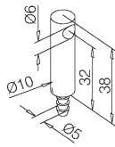
Eindsteun - 660 / 06
