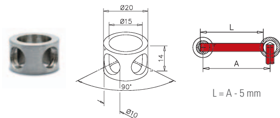
692 / 10 - voor hoeksteun 90°
