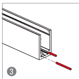
Centreer-koppel stift Art.Nr. 93.1010.330.00 (121)
