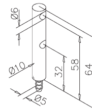
Dubbele middensteun - 666 / 06
