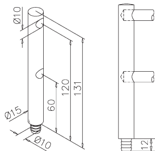
Dubbele eindsteun - 665 / 10
