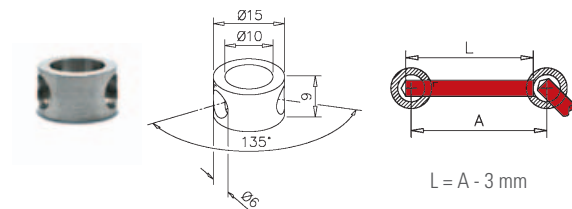
693 / 06 - voor hoeksteun 45°
