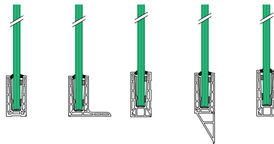
Easy Glass® Pro Montage au sol / Scellement béton Easy Glass® Pro F Montage au sol Easy Glass® Pro Montage latéral Easy Glass® Pro Y Montage latéral Easy Glass® Pro Inverse Montage latéral
