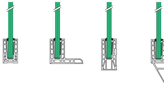
Easy Glass® Max Montage au sol / Scellement béton
